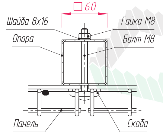
Б-Б (Увеличено)
